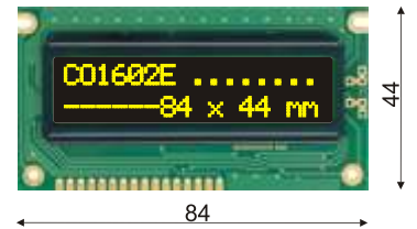
CO-1602E (16Chr. x 2 Lines)
